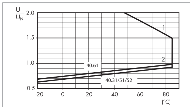
R 40 - Campo de funcionamiento de la bobina DC en función de la temperatura ambiente - Bobina sensible, tipos 40.31/51/52/61
