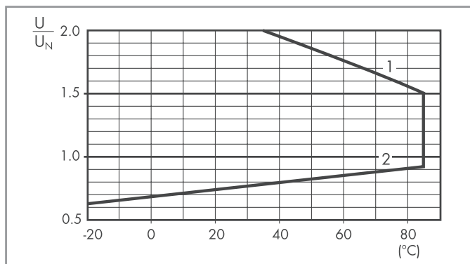
R 40 - Campo de funcionamiento de la bobina DC en función de la temperatura ambiente - Bobina estándar
