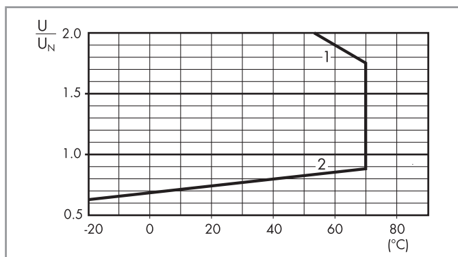
R 40 - Campo de funcionamiento de la bobina DC en función de la temperatura ambiente - Bobina sensible, tipo 40.11
