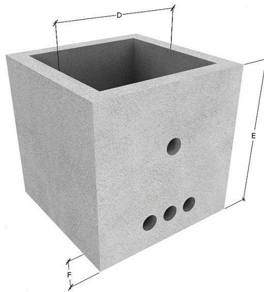
ISOMETRICO
