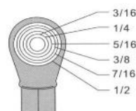
CALIBRE 2 AWG
