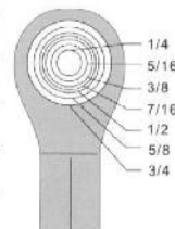
CALIBRE 1/0 AWG
